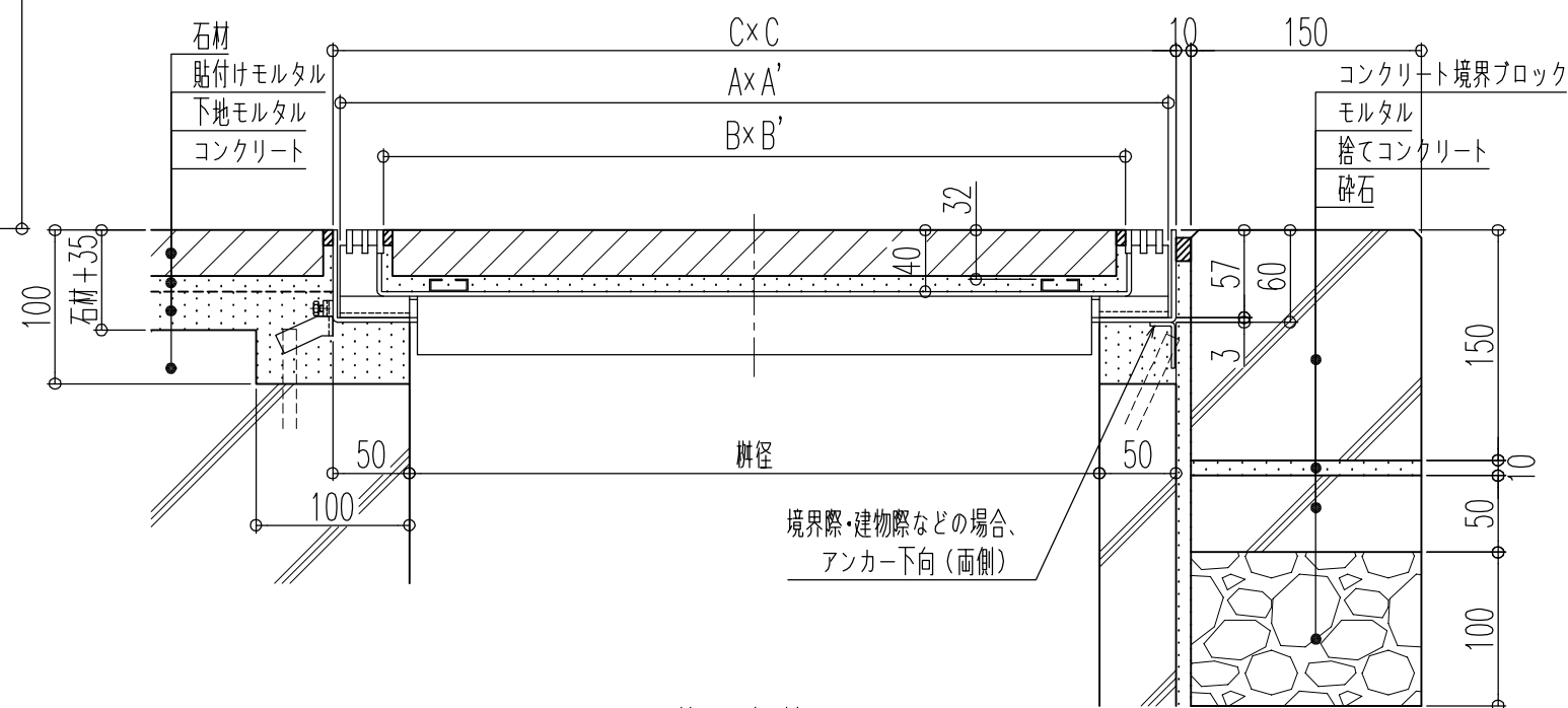
施工参考图
